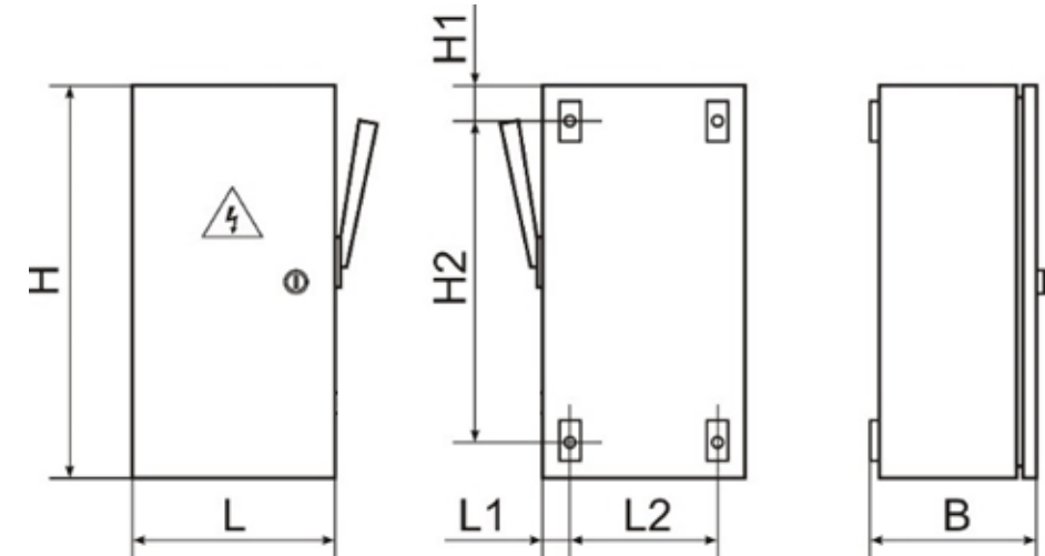
Рисунок 1. Общий вид и габаритные размеры ЯРП11М-3
