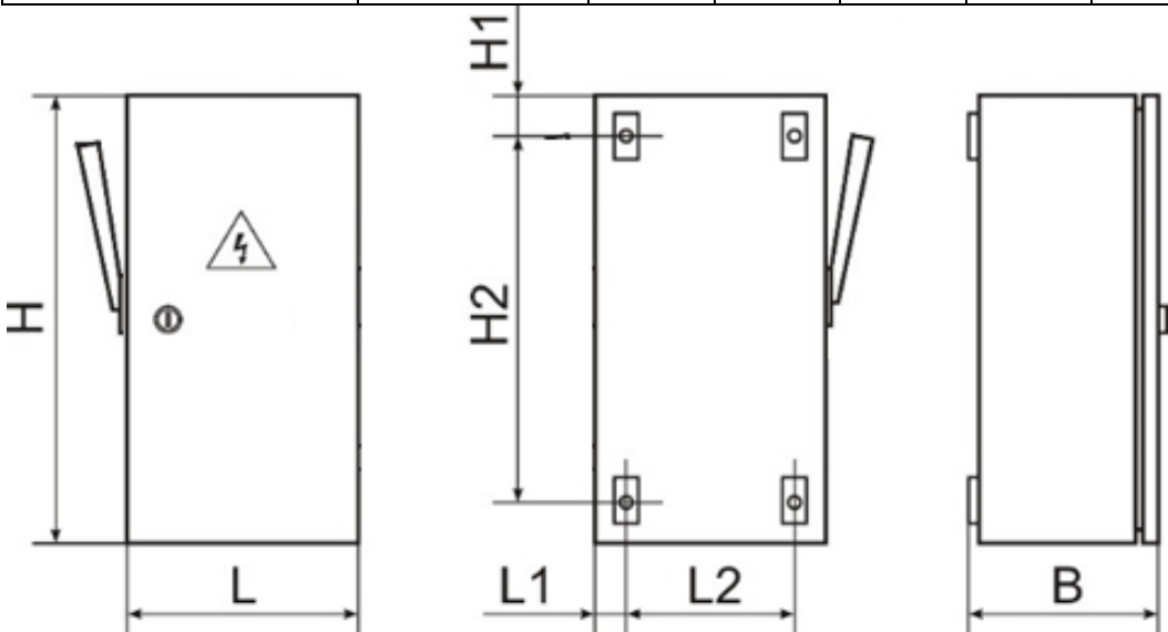
Рисунок 3. Общий вид и габаритные размеры ЯРП11М-7
